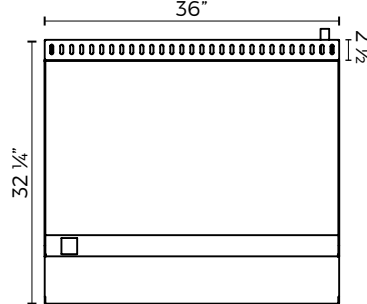
AEMG-36 (H) TOP
